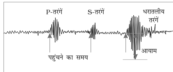
चित्र 3.1 : भूकंप-अभिलेख
