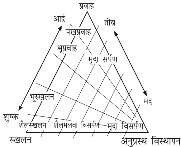
चित्र 6.5 : वृहद् संचलन के विभिन्न रूपों का सह-संबंध, उनकी सापेक्ष गति की दर एवं आर्द्रता की सीमा (क्वाइटहेड, 2001)
