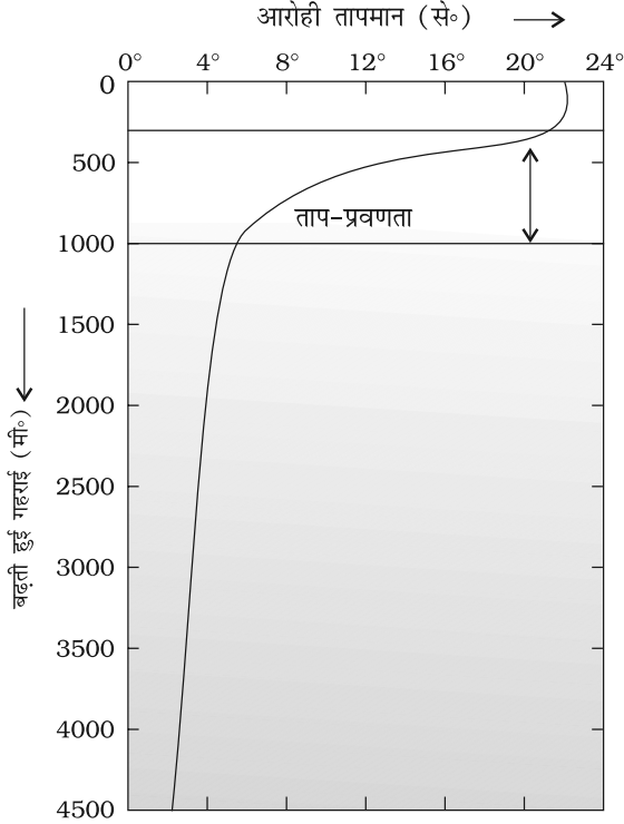
चित्र 13.3 : ताप प्रवणता (थर्मोक्लाइन)
